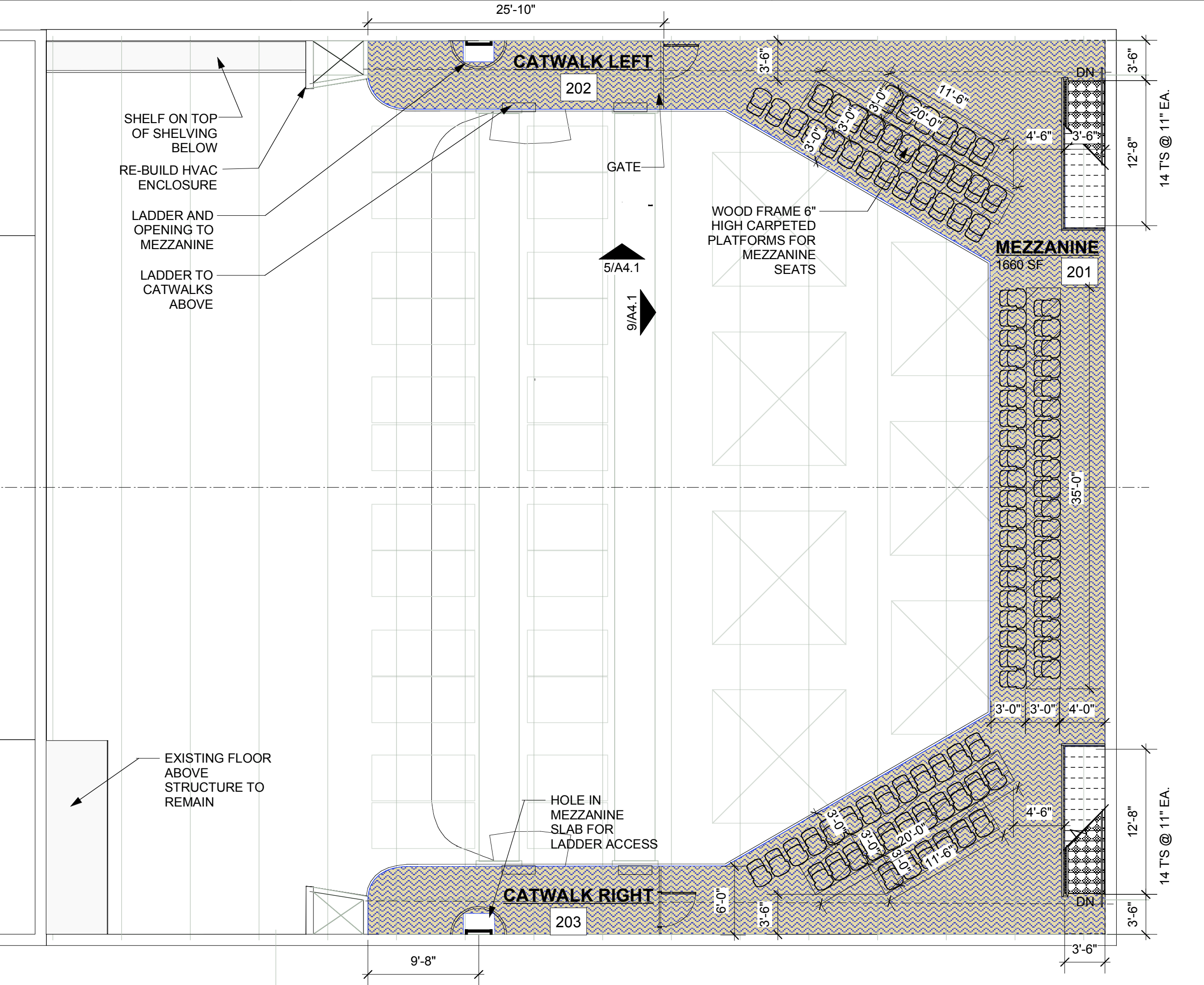
1 MEZZANINE PLAN A1.2 Scale: 1/8" = 1'-0"
